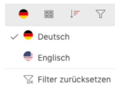
Abbildung 73: Filter zurücksetzen
