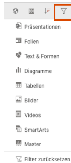
Abbildung 54: Filter
