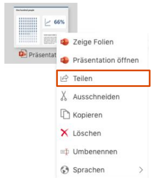
Abbildung 77: empower ® Link
