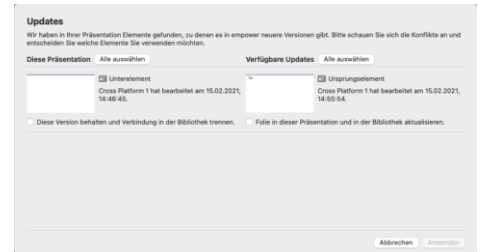
Abbildung 90: Update Wizard
