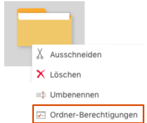
Abbildung 50: Ordner-Berechtigungen anzeigen
